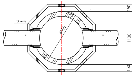
平面図
