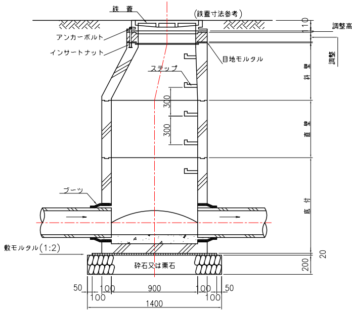
縦断面図
