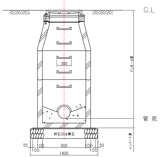
横断面図
