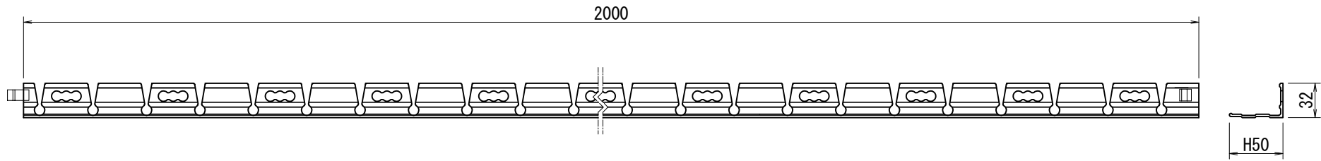
スパイク (釘) S=1:5
