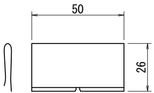
連結用クリップ S=1:2
