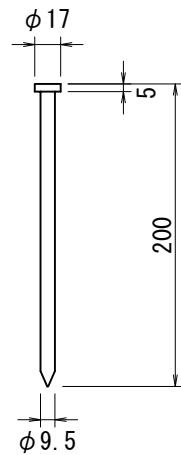
スパイク (釘) S=1:5
