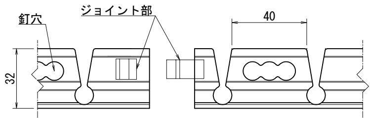
連結部拡大図 S=1:2
