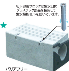
バリアフリー 0～2cm段差
