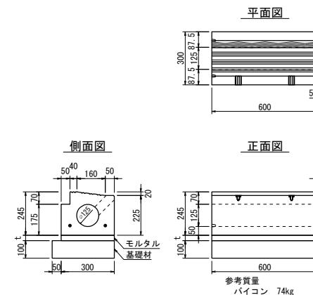
【参考図】 ライン導水ブロックF型 構造図 歩道切下 バリアフリー 直線 VP
