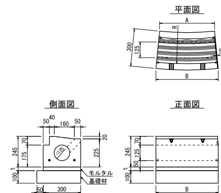
【参考図】 ライン導水ブロックF型 構造図 歩道切下 バリアフリー 曲線
