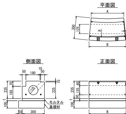
【参考図】 ライン導水ブロックF型 構造図 歩道切下 フラット1CM 曲線
