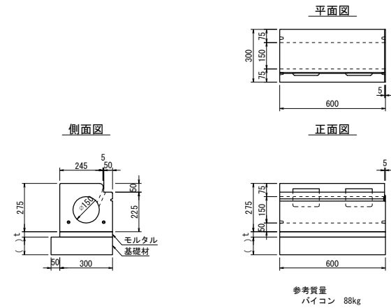
【参考図】 ライン導水ブロックF型 構造図 車両乗入 フラット5CM N
