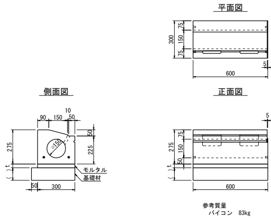
【参考図】 ライン導水ブロックF型 構造図 車両乗入 テーパー N
