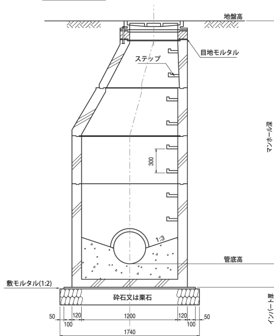
横断面図
