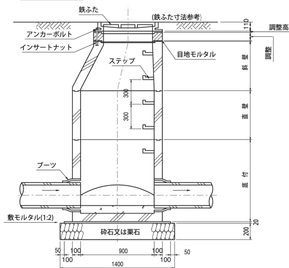
縦断面図
