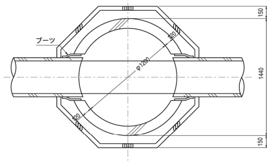
縦断面図
