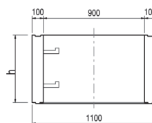
直壁 VMS1
