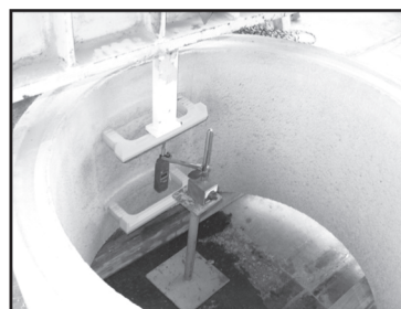
垂直方向荷重試験(歪み5.4mm)
