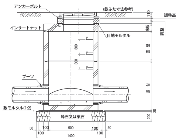
縦断面図
