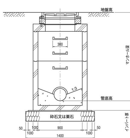
横断面図
