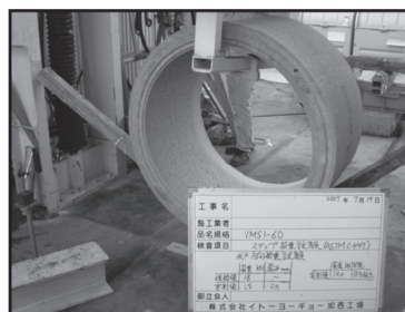
水平方向荷重試験(異常なし)
