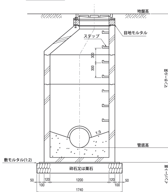
横断面図
