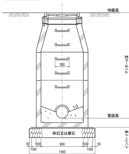
横断面図
