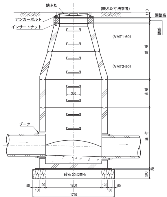
縦断面図
