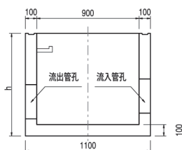
底付 VMB1 (管取付壁)
