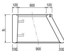
斜壁 VMT1
