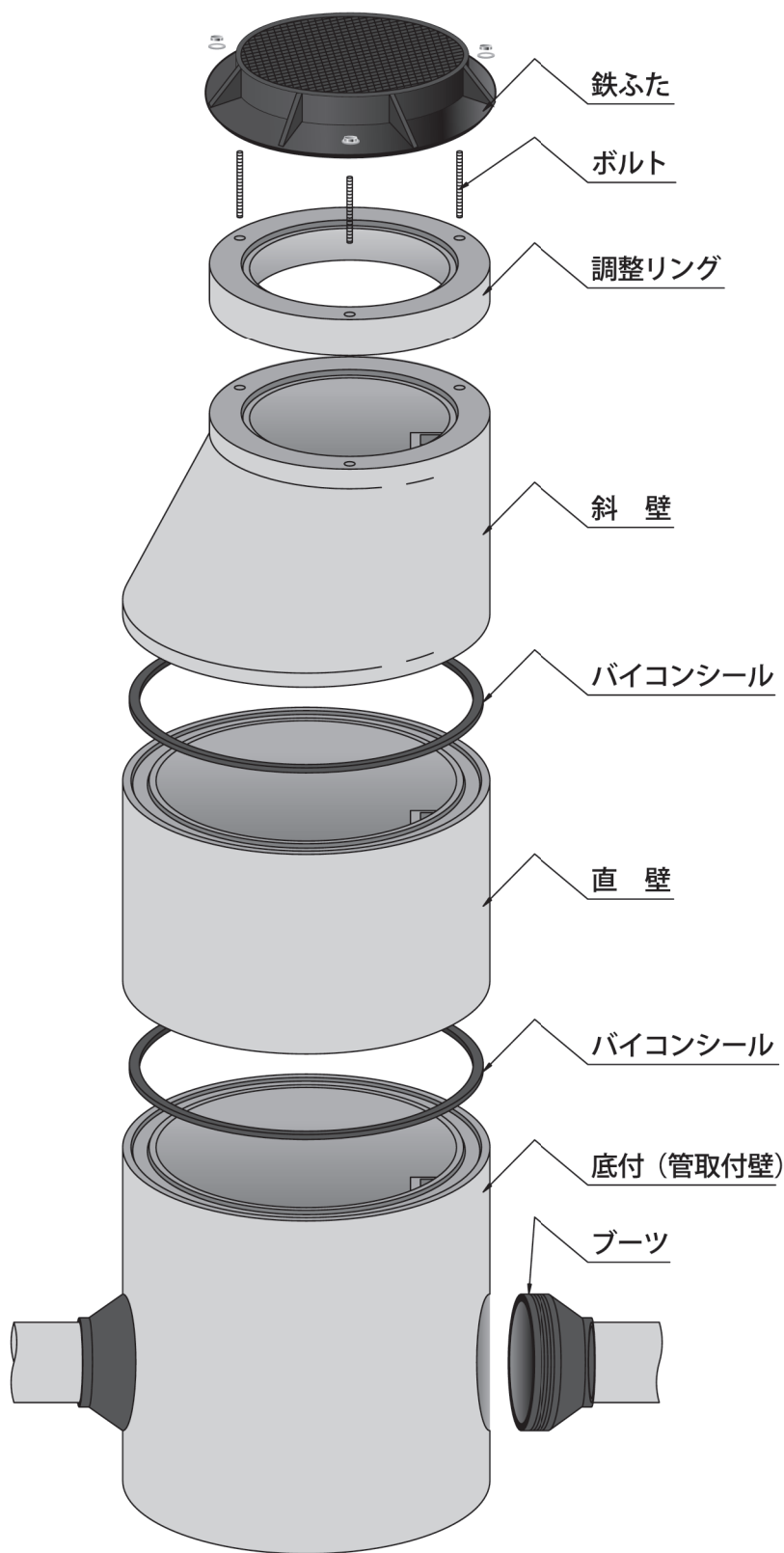
組立図
