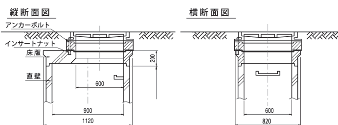
床版ブロック使用の場合
