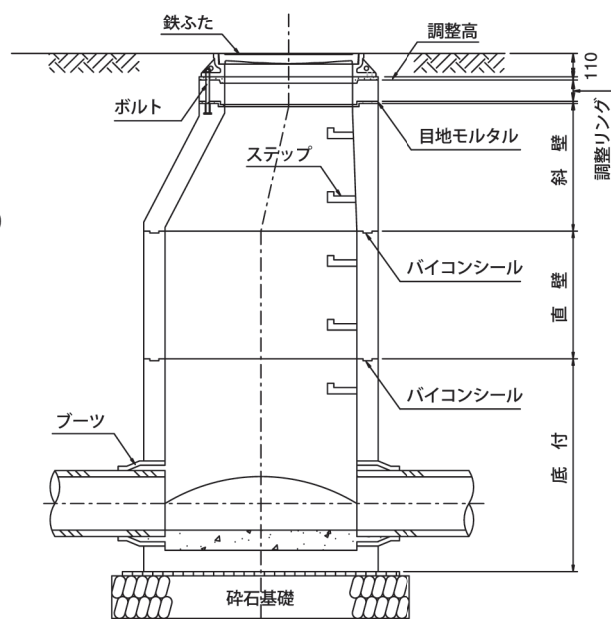
組立図
